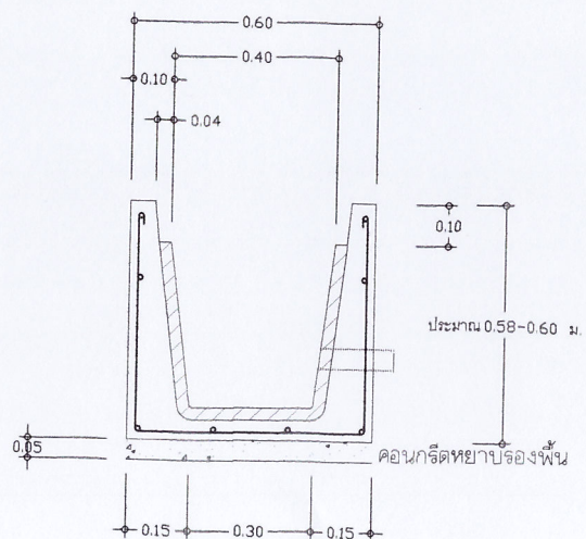
รูปตัดตามขวาง I: 20
