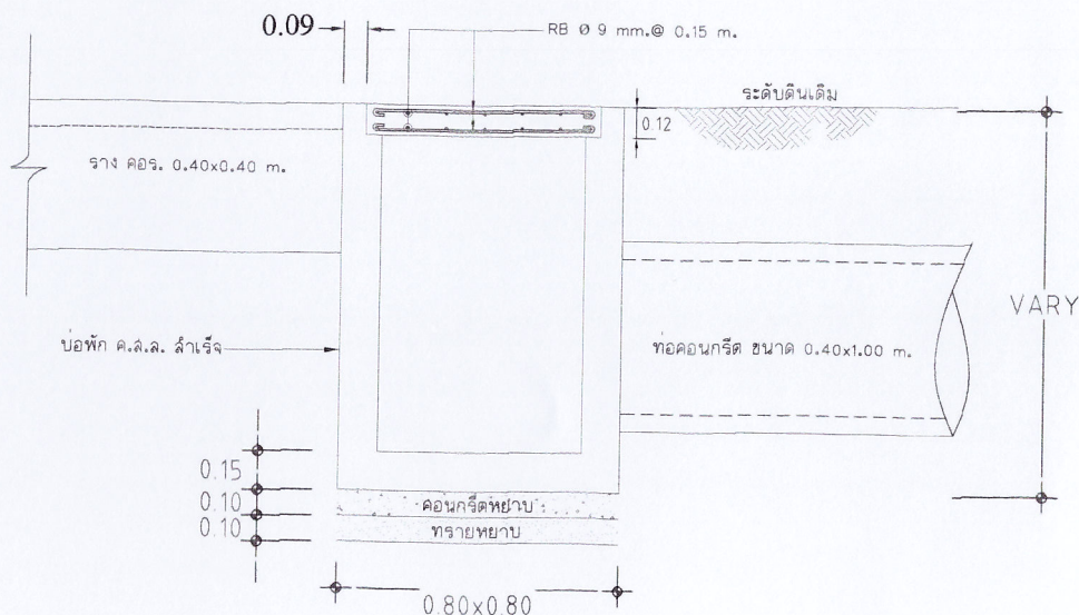
รูปด้าน Not to Scale
